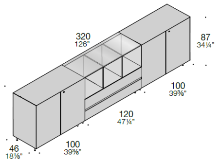
Container L320 (1 W120 module + 2 W100 modules)
