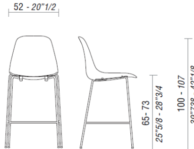
POLA, sgabello con 4 gambe in metallo.
