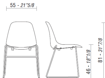
POLA, sedia con base a slitta lineare.
