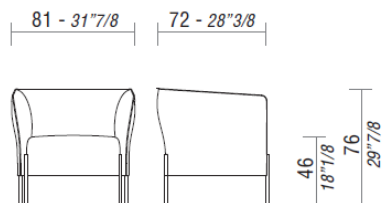
DOLLY, poltrona H76.
