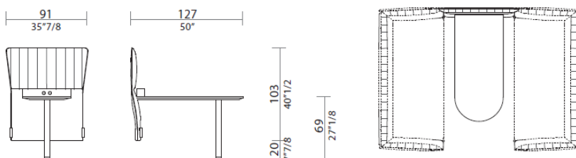
Pannello tecnico Dolly Chat con tavolo.
