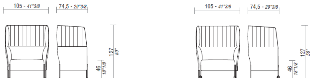
DOLLY, poltrona Eremo con e senza ruote.
