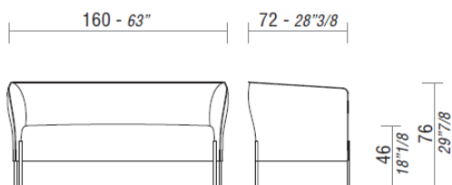
DOLLY, divano H76.
