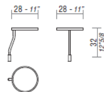
\phi 28 cm Laccato, sp 2cm.
