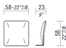
DOLLY, schienale per panca.
