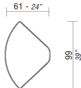
DOLLY, raccordo tavolino 90°.
