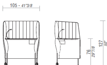
DOLLY DESK, con tavolino integrato.
