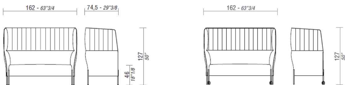
DOLLY, divano Chat con e senza ruote.
