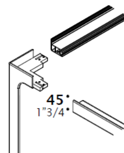
Dettaglio struttura
