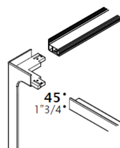
Dettaglio struttura
